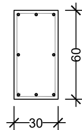
PENULANGAN BALOK INDUK 30 X 60
