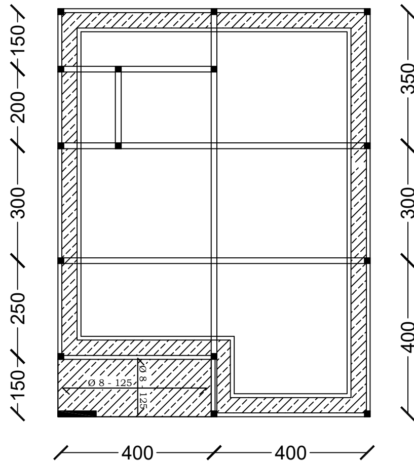
DENAH RING LT2 SKALA 1 : 100
