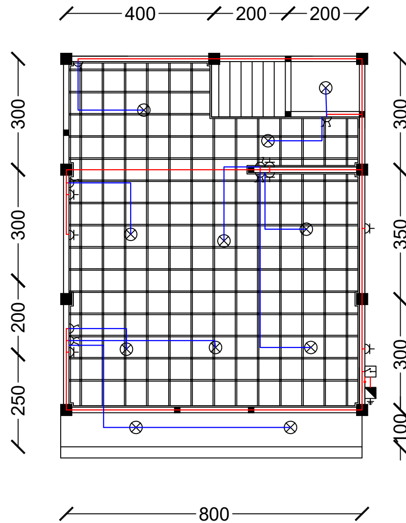
PLAFON & KELISTRIKAN LT 1 SKALA 1 : 100
