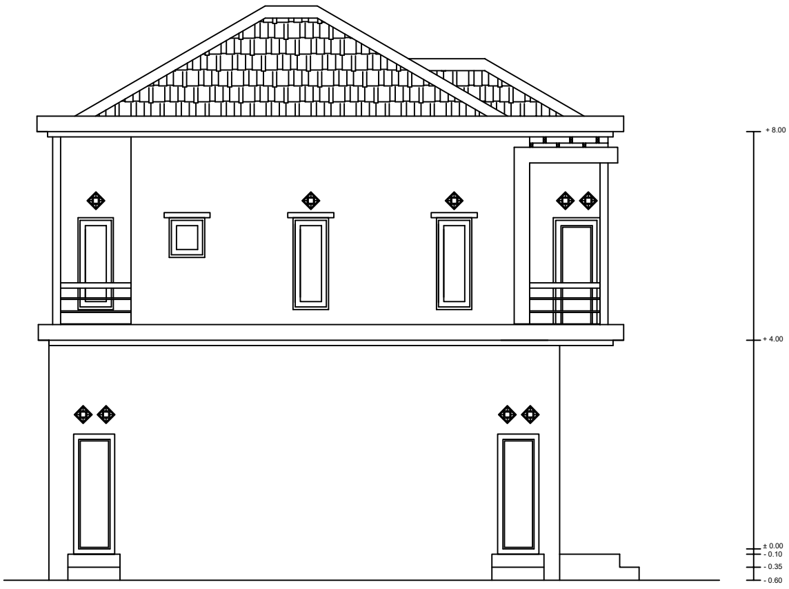
SAMPING KANAN SKALA 1 : 100
