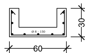
PENULANGAN TALANG BETON
