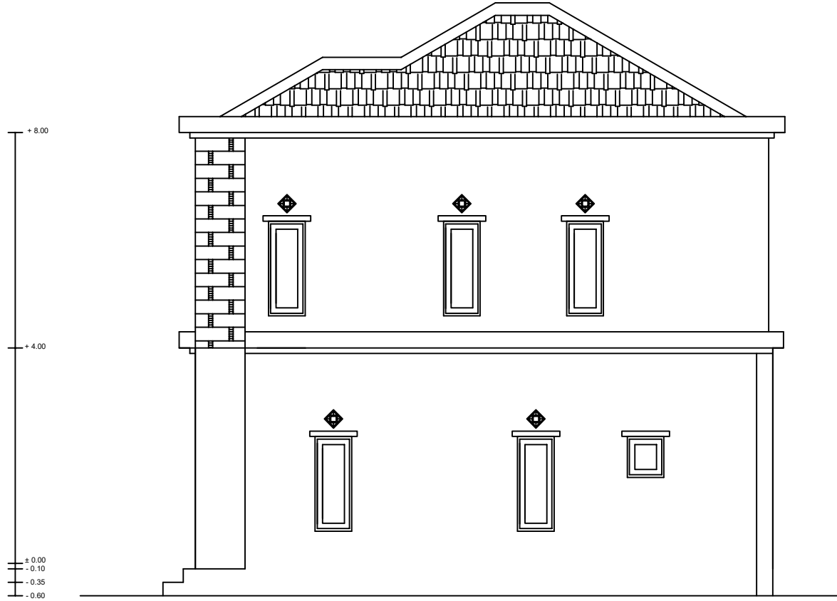
SAMPING KIRI SKALA 1 : 100
