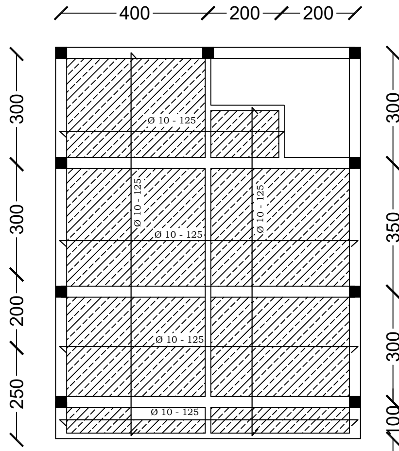
DENAH BETON LT2 SKALA 1 : 100
