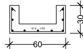
PENULANGAN TALANG BETON
