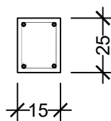
PENULANGAN BALOK ANAK & RING 15 X 25
